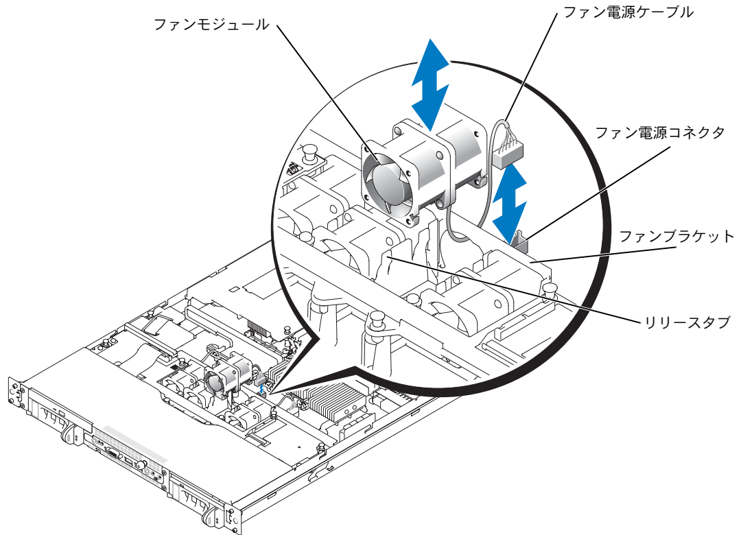
図 1. ファンモジュールの取り外しと取り付け
